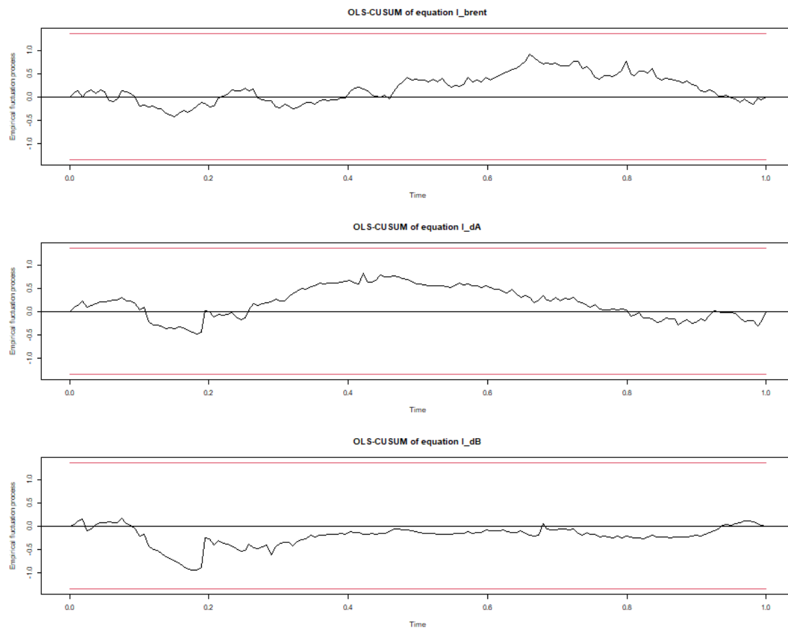
Figura 4: Gráficos OLS-CUSUM para as três equações do sistema. As linhas vermelhas são as bandas de confiança a 5%.
